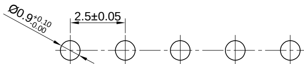
P.C.B LAYOUT
