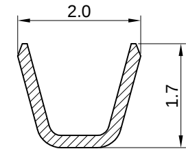
SEC D-D
